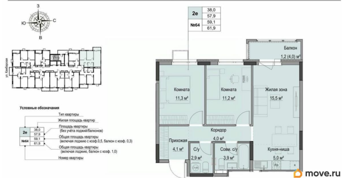
Секция № 1. План квартиры № 64 на 8 этаже
