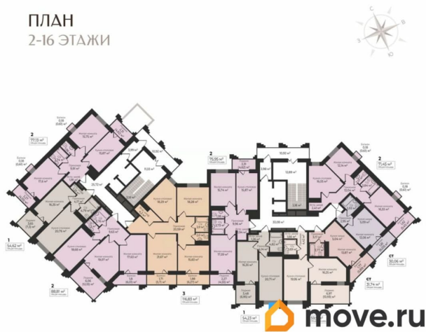
2-16 ЭТАЖИ
