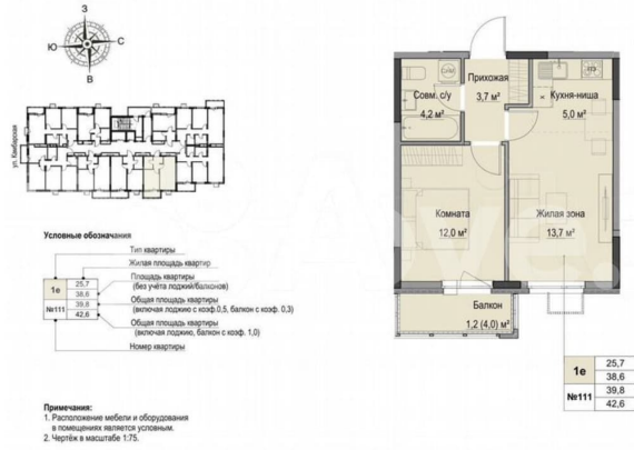
Многоквартирный жилой комплекс (Дом №1, Дом №2) на улице Камбарская, город Ижевск 2 этап строительства. Жилой дом №2
