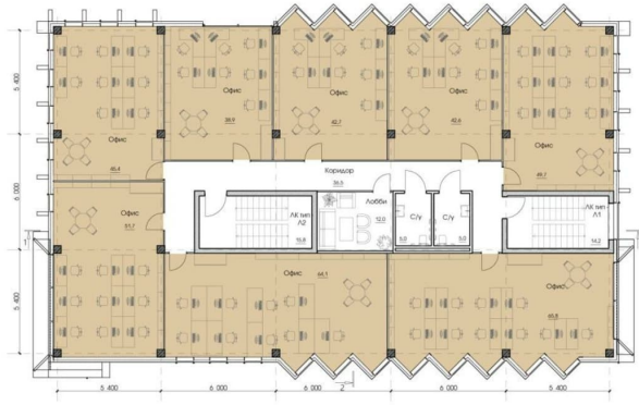
План 2 этажа
